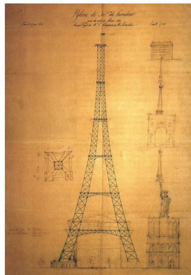
2 Eiffelova veža v Paríži. Návrh: Alexander Gustave Eiffel, realizácia: Gustave Eiffel & Cie. Železné diely. Francúzsko, 1889
